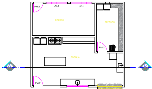
PLANTA BAIXA ESCALA 1/100
