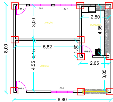
PLANTA BAIXA ESCALA 1/100
